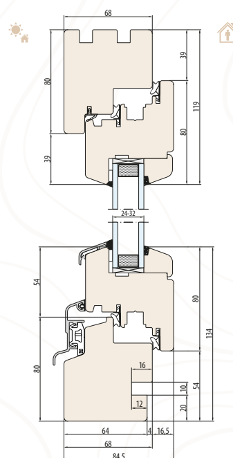
SISTEMA NATURO 68 Scanalatura per davanzale interno
