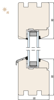
SISTEMA NATURO 68-FIX Senza scanalatura per il davanzale
