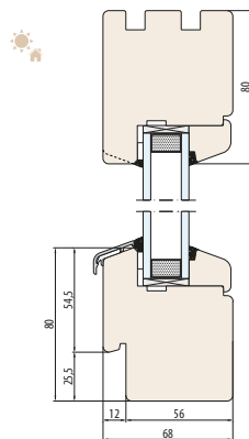
SISTEMA NATURO 68-FIX Scanalatura per davanzale esterno
