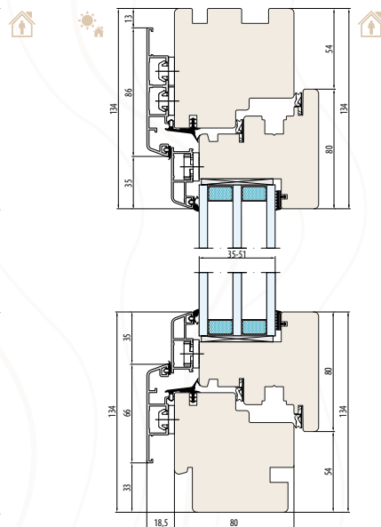
SISTEMA NATURO 80 ALU GEMINI CLASSIC Scanalatura per davanzale interno ed esterno
