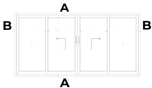
SISTEMA NATURO 68 HST (Dimensioni generali) - soglia 22 mm - schema "C"
