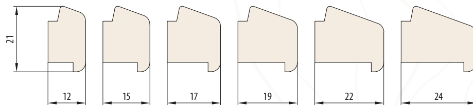
LISTELLO FERMAVETRO RETRÒ
