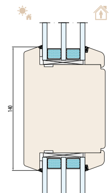
SISTEMA NATURO 92 szpros konstrukcyjny 140 mm
