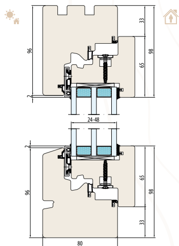
SISTEMA ESPERIA LIFE 80 Senza scanalatura per il davanzale
