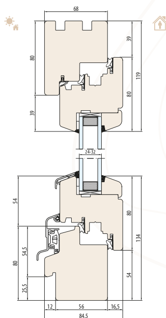
SISTEMA NATURO 68 Scanalatura per davanzale esterno
