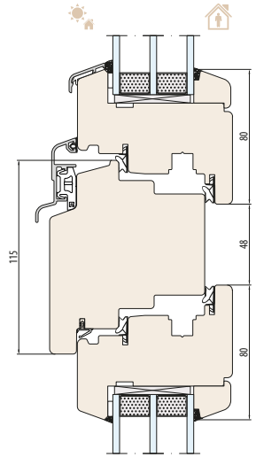
SISTEMA NATURO 92 slėmių 115 mm
