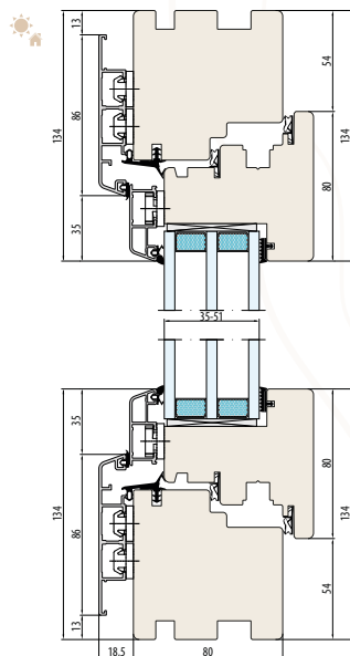
SISTEMA NATURO 80 ALU GEMINI CLASSIC Senza scanalatura per il davanzale
