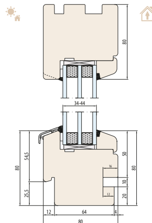
SISTEMA NATURO 80-FIX Scanalatura per davanzale interno ed esterno
