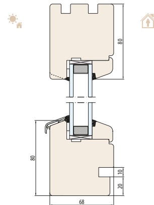
SISTEMA NATURO 68-FIX Scanalatura per davanzale interno
