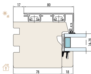
SISTEMA ESPERIA LIFE 74 ALU-Fix SEZIONE ORIZZONTALE B-B
