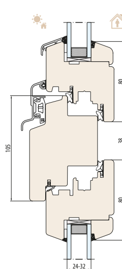
SISTEMA NATURO 68 Traverso 105 mm
