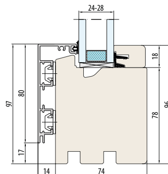
SISTEMA ESPERIA LIFE 74 ALU-Fix Senza scanalatura per il davanzale
