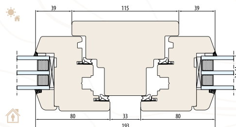
SISTEMA NATURO 80 Montante fisso 115 mm (Sezione orizzontale)
