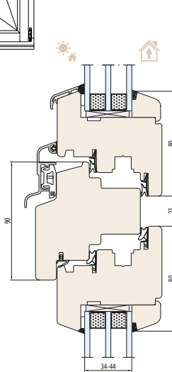
SISTEMA NATURO 80 Traverso 90 mm
