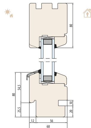
SISTEMA NATURO 68-FIX Scanalatura per davanzale interno ed esterno
