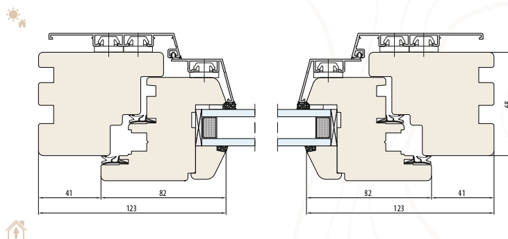
SISTEMA NATURO 68 ALU RENO LINE
