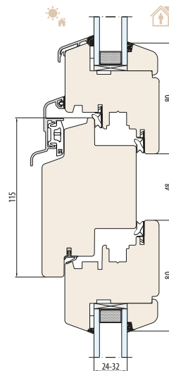
SISTEMA NATURO 68 Traverso 115 mm
