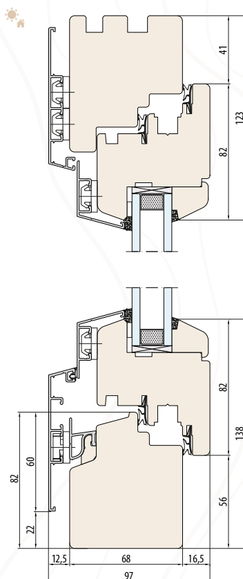
SEZIONE VERTICALE A-A
