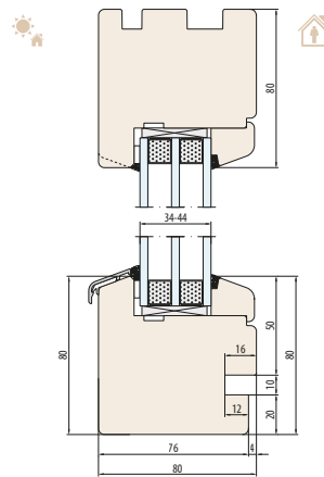
SISTEMA NATURO 80-FIX Scanalatura per davanzale interno
