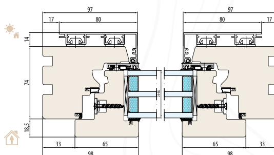
SISTEMA ESPERIA LIFE 74 ALU SEZIONE ORIZZONTALE B-B
