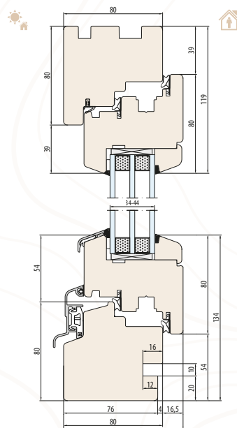
SISTEMA NATURO 80 Scanalatura per davanzale interno
