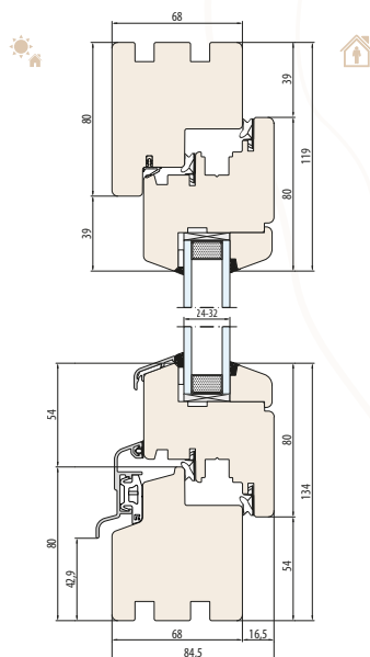
SISTEMA NATURO 68 Senza scanalatura per il davanzale
