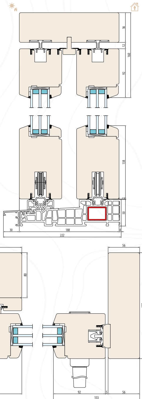
SISTEMA NATURO 80 HST (Dimensioni generali) - soglia 50 mm - schema "D"
