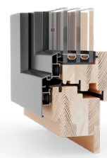
Gemini Classic Profilo di ristrutturazione (con scanalatura)
