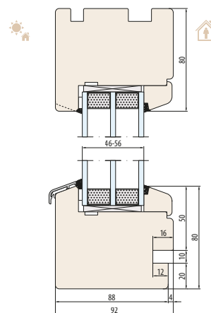
SISTEMA NATURO 92-Fix Scanalatura per davanzale interno
