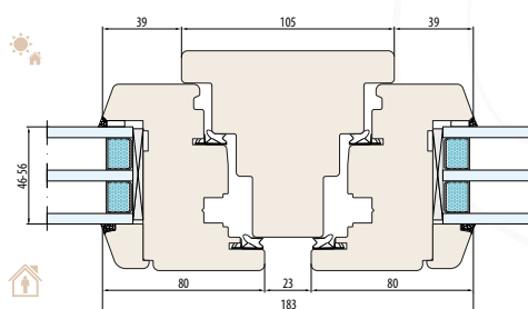
SISTEMA NATURO 92 Montante fisso 105 mm (Sezione orizzontale)
