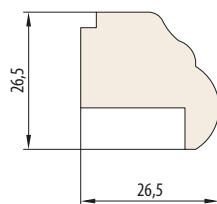
LISTELLO FERMAVETRO SOVRAPPOSTO
