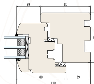
SISTEMA NATURO 80 Scanalatura per davanzale interno
