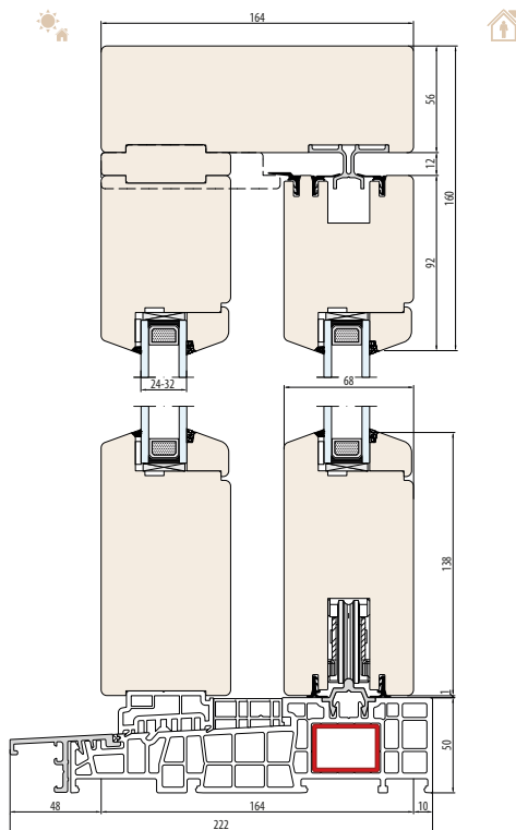
SISTEMA NATURO 68 HST (Dimensioni generali) - soglia 50 mm - schema "C"
