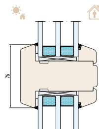
SISTEMA NATURO 92 szpros konstrukcyjny 76 mm
