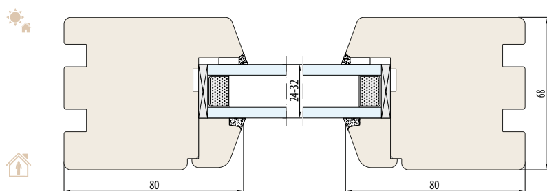
SISTEMA NATURO 68-FIX SEZIONE ORIZZONTALE B-B
